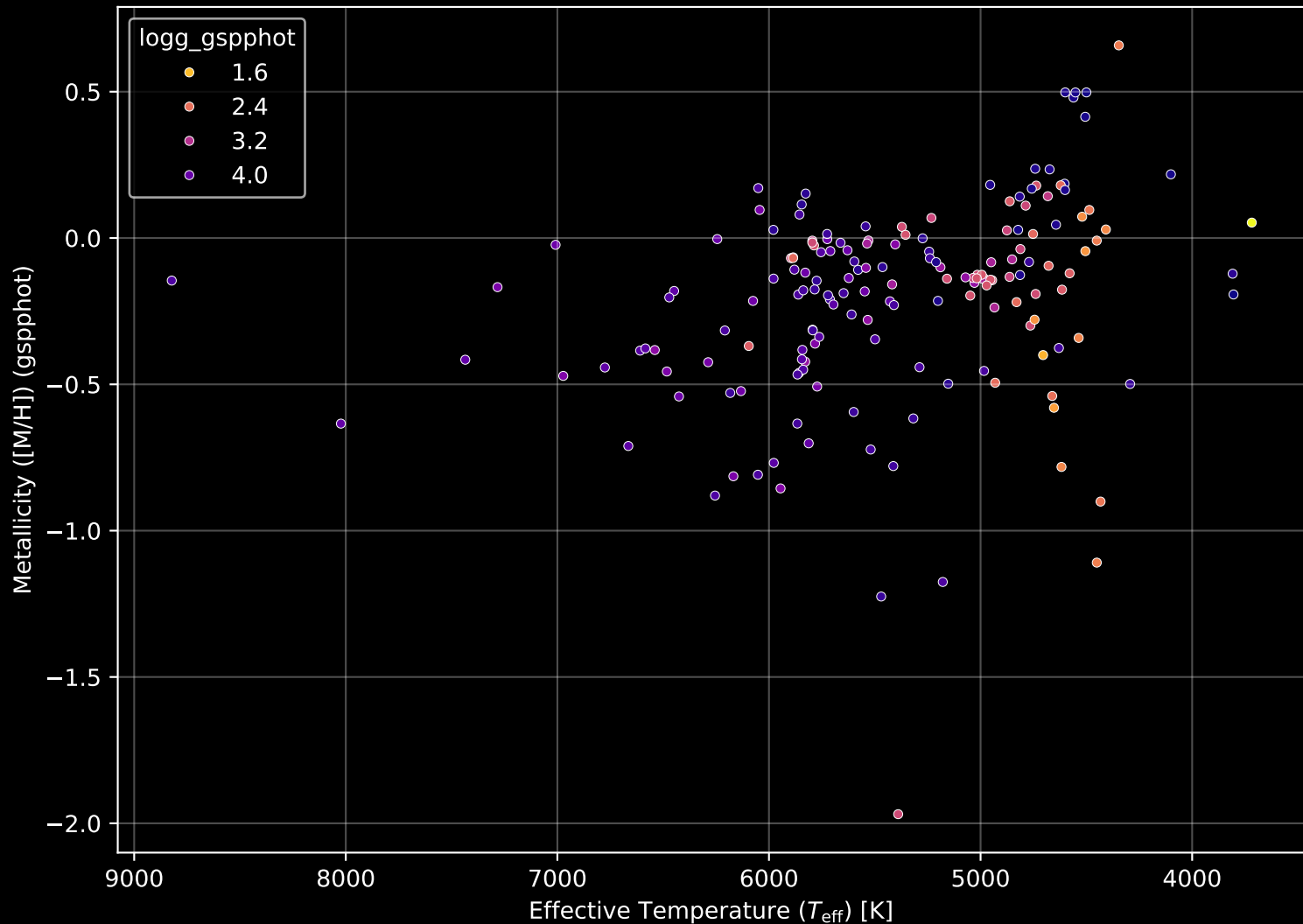
APOGEE DR17 Field: [286-29-O_TESS] Stellar Population Parameters (n= 172)
