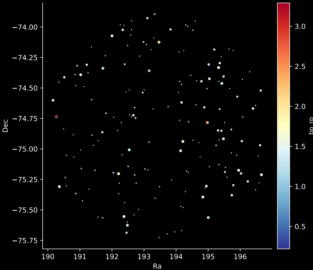
APOGEE DR17 Field: [286-29-O_TESS] Stars: 172
